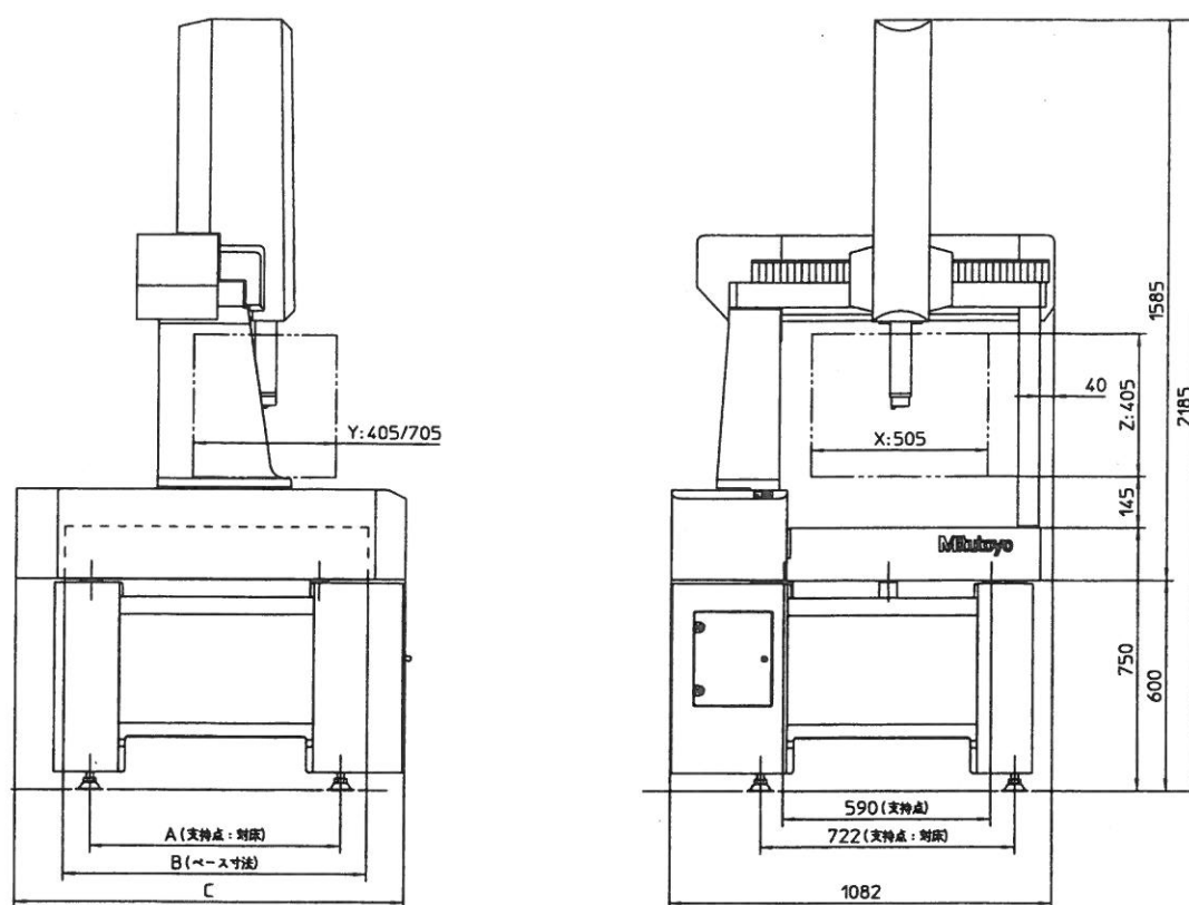
外観寸法図 (単位:mm)
