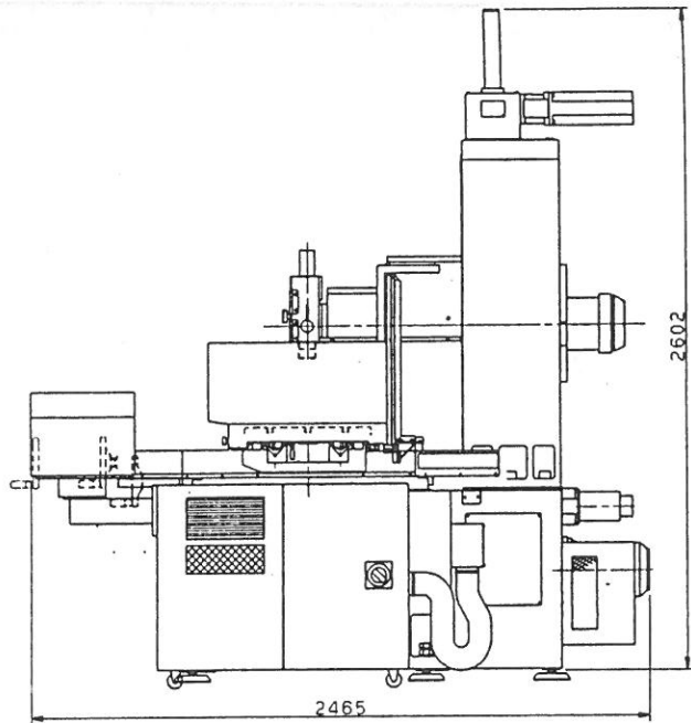
外形図
