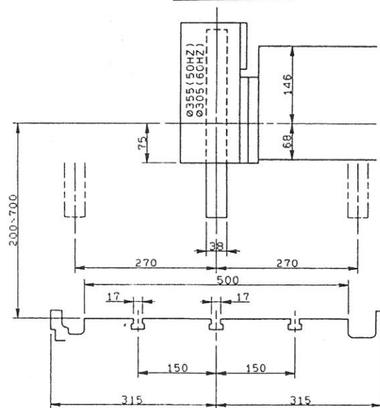
加工範囲図
