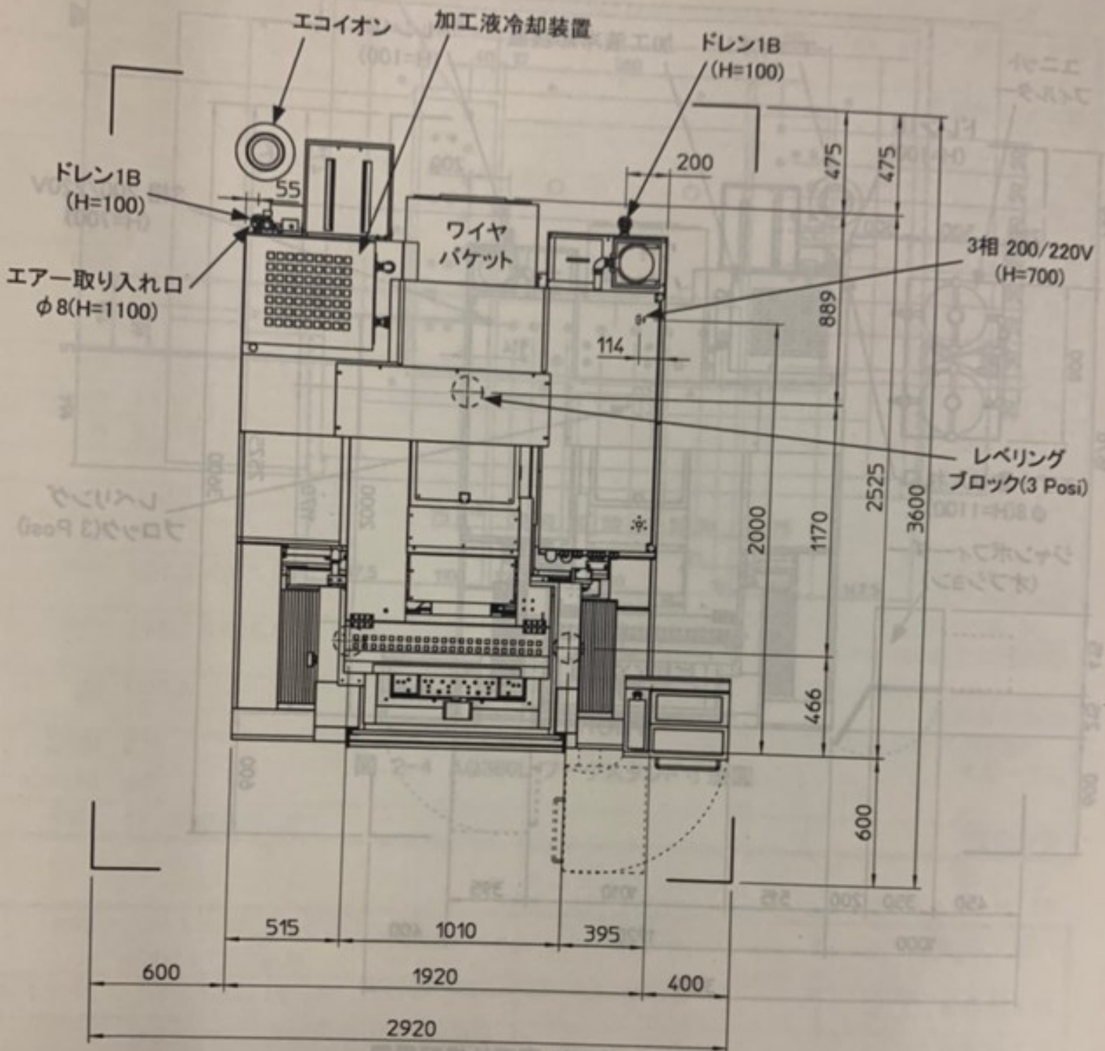
図 2-2 AQ360L 配置図
