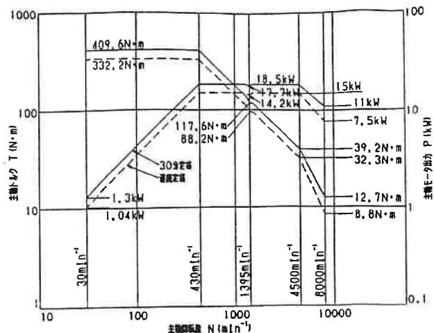
図2.1 主軸N-T, N-P特性 (AC15/18.5KW)
