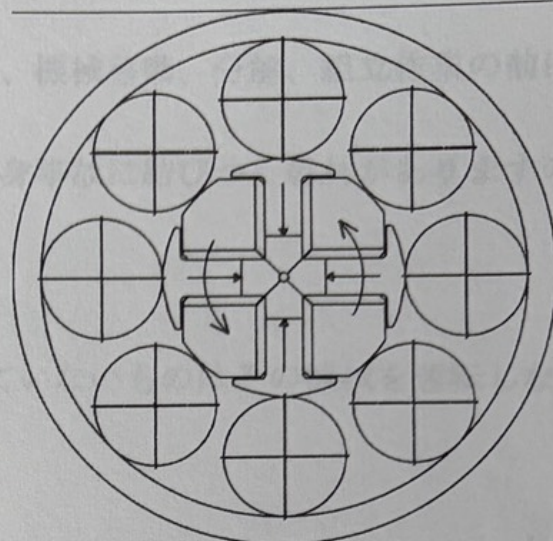
加圧状態（閉じる）
