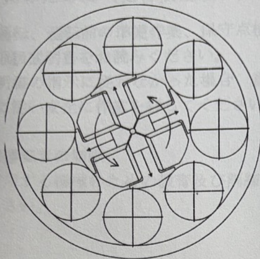
非加圧状態（開く）
