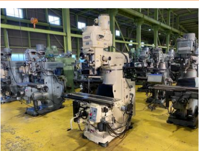
ラム型フライス 牧野フライス KVJP-55 1993年製 管理番号:H016571 置場:マシンプラザ本庄
