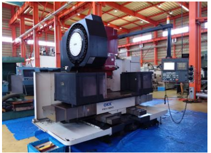
立型マシニングセンター OKK MCV-560 2006年製 FANUC160is-MB BT50 管理番号:P008103 置場:東日本マシンブラザ
