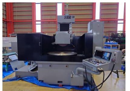
横軸ローラー研削盤 住友重機械 SHR-110 1996(2023年7月0/H)年 FANUC0-M テーブルサイズφ1100 管理番号:P008097 置場:東日本マシンプラザ
