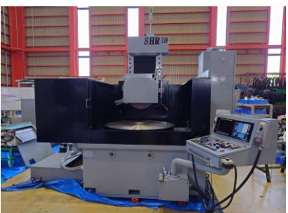
横軸ロータリー研削盤 住友重機 SHR-110 1996(2023年7月O/H)年 FANUC0-M テーブルサイズ'φ1100 管理番号:P008097 置場:東日本マシンブラザ
