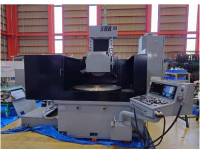
横軸ロータリー研削盤 住友重機 SHR-110 1996(2023年7月O/H)年 FANUC0-M テーブルサイズ'φ1100 管理番号:P008097 置場:東日本マシンプラザ
